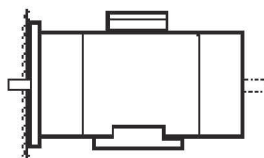
IM2081(IM2082) большой фланец *IM B34 большой фланец IM2181(IM2182) малый фланец *IM B35 малый фланец
