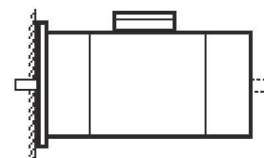
IM3041(IM3042) большой фланец *IM B5 большой фланец IM3641(IM3642) малый фланец *IM B9 малый фланец
